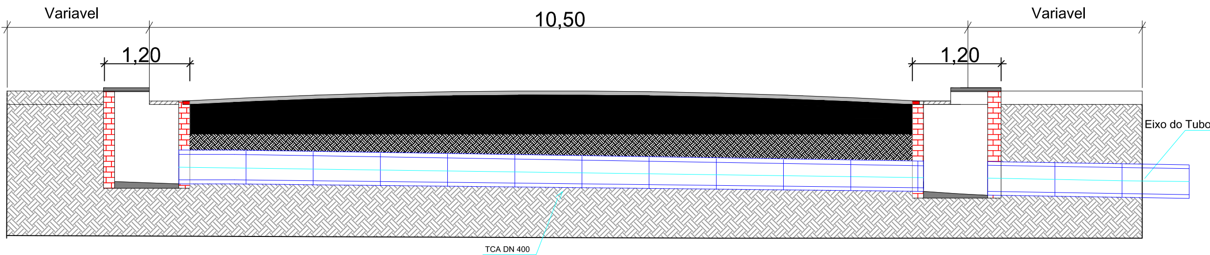
Corte A' A'
