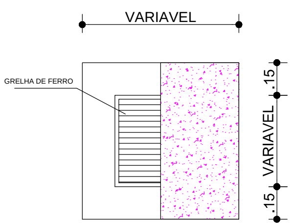
BOCA DE LOBO PLANTA BAIXA ESCALA: 1/25
