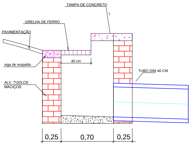
CORTE AB ESCALA: 1/25
