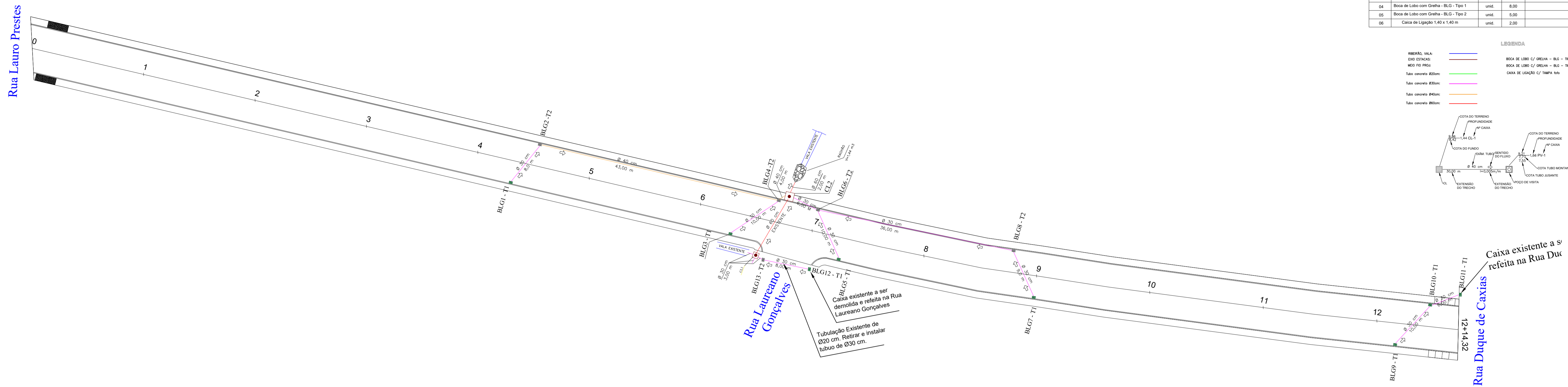
PLANTA BAIXA DE IMPLANTAÇÃO - REDE DE DRENAGEM Sem Escala
