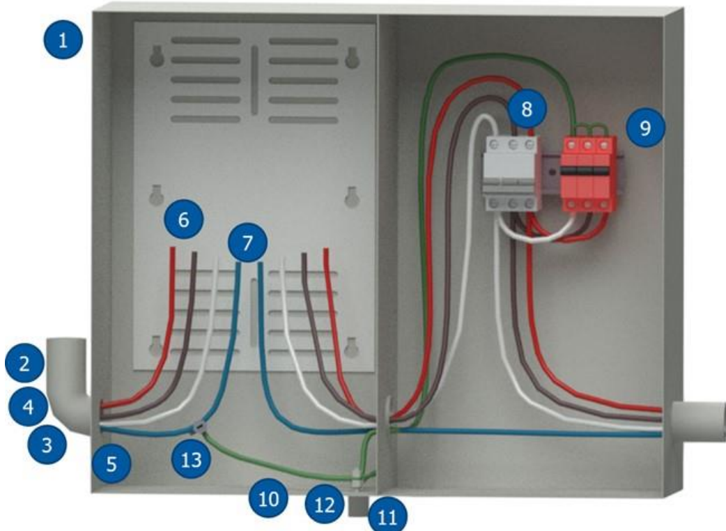
Figura 12 - Ligação Trifásica
