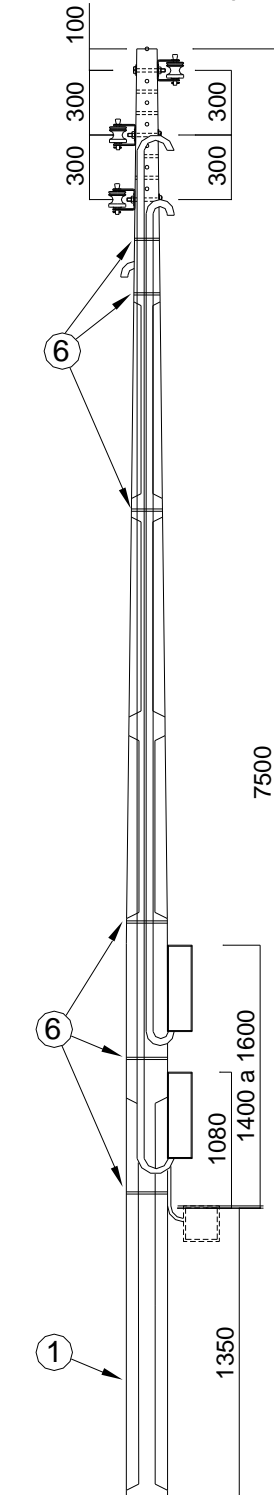
Vista Lateral Esquerda
