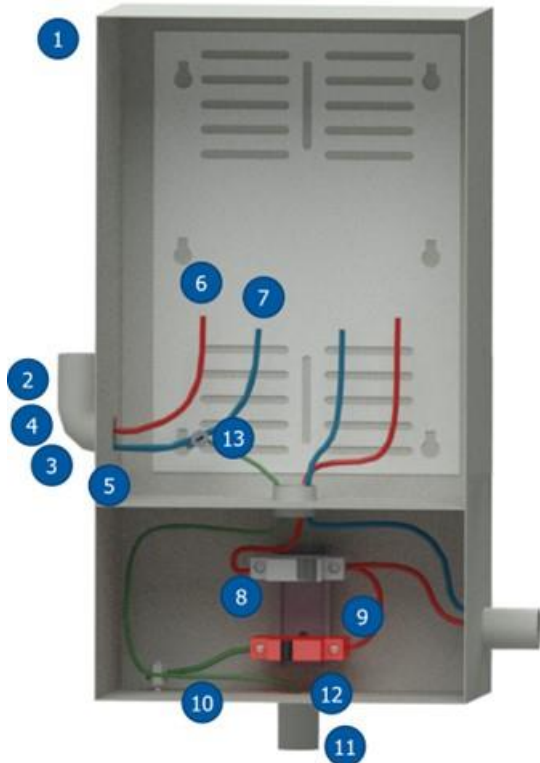
Figura 10 - Ligação Monofásica
