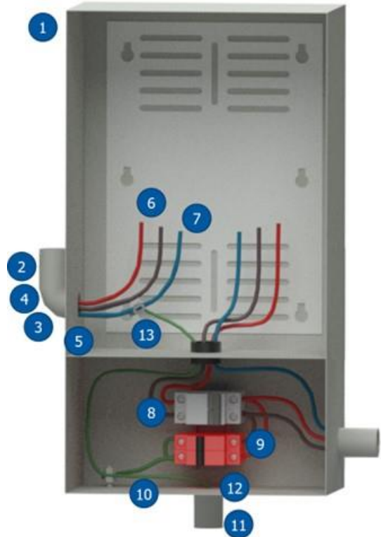
Figura 11 - Ligação Bifásica
