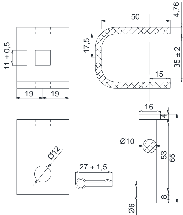
Estribo
