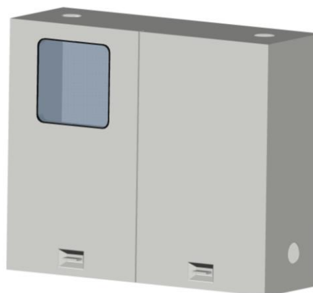
Figura 7 - Caixa Tipo III - Ligações Trifásicas com medição direta
