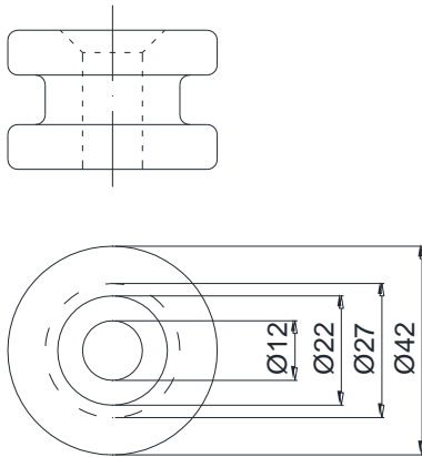
Isolador
