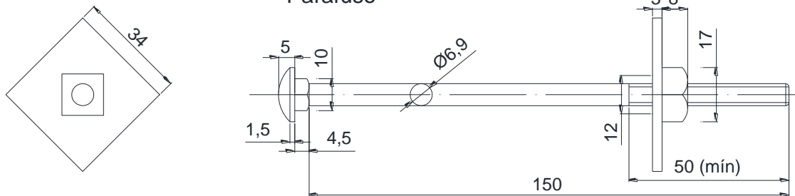
Parafuso
