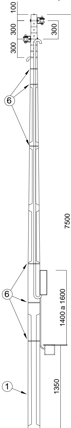
Vista Lateral Esquerda
