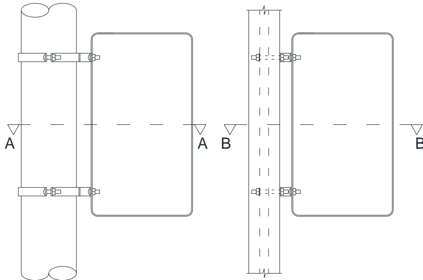
Caixa em poste circular de aço
