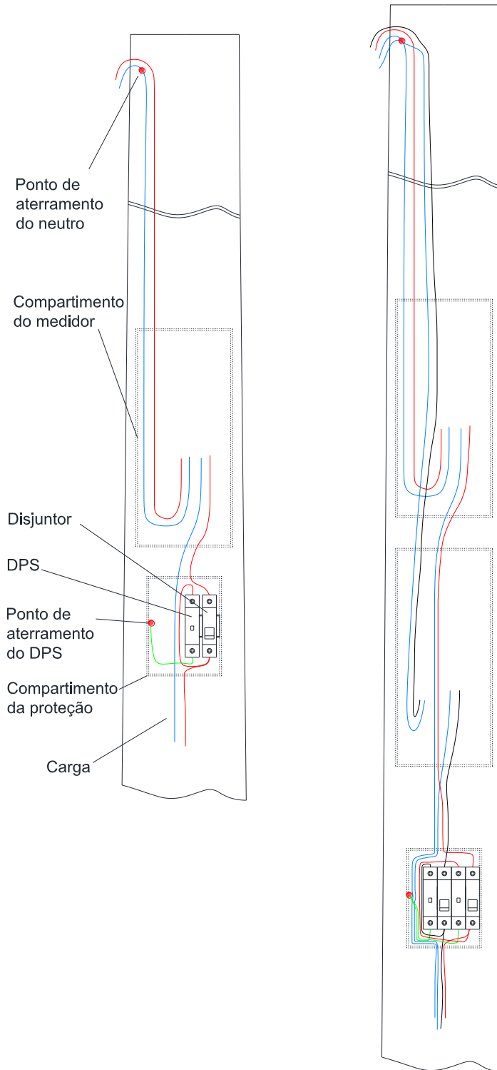
Poste de concreto auto aterrado.
