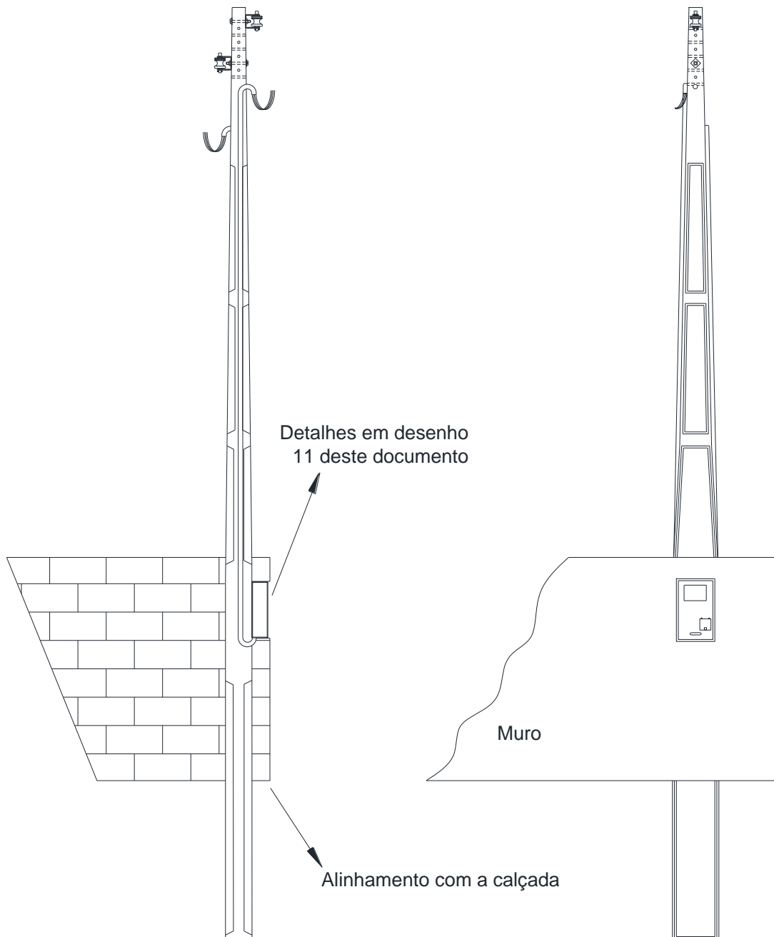
Vista Lateral
