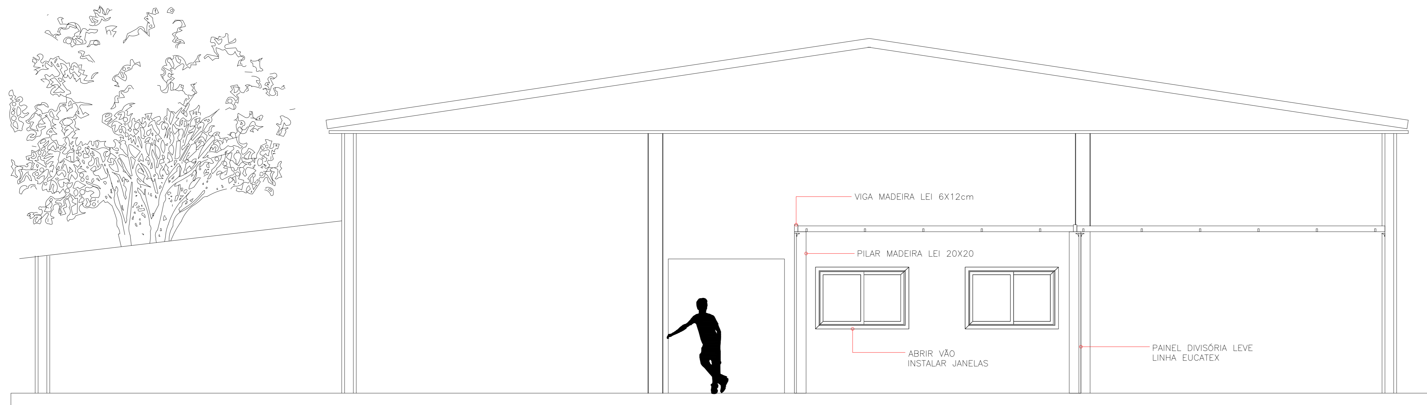
01 CORTE BB ESC.1:100
